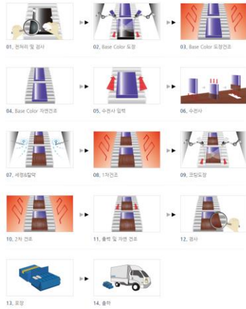
그림 3. Curl-Fit 공정과정
